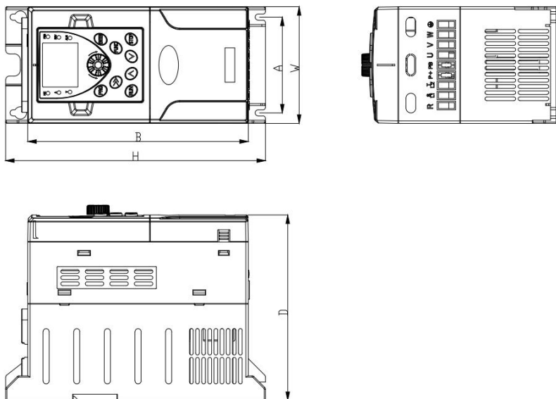
图 D-1 变频器 1.5KW~22KW 尺寸
