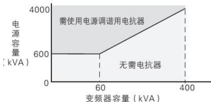
电抗器的安装条件
