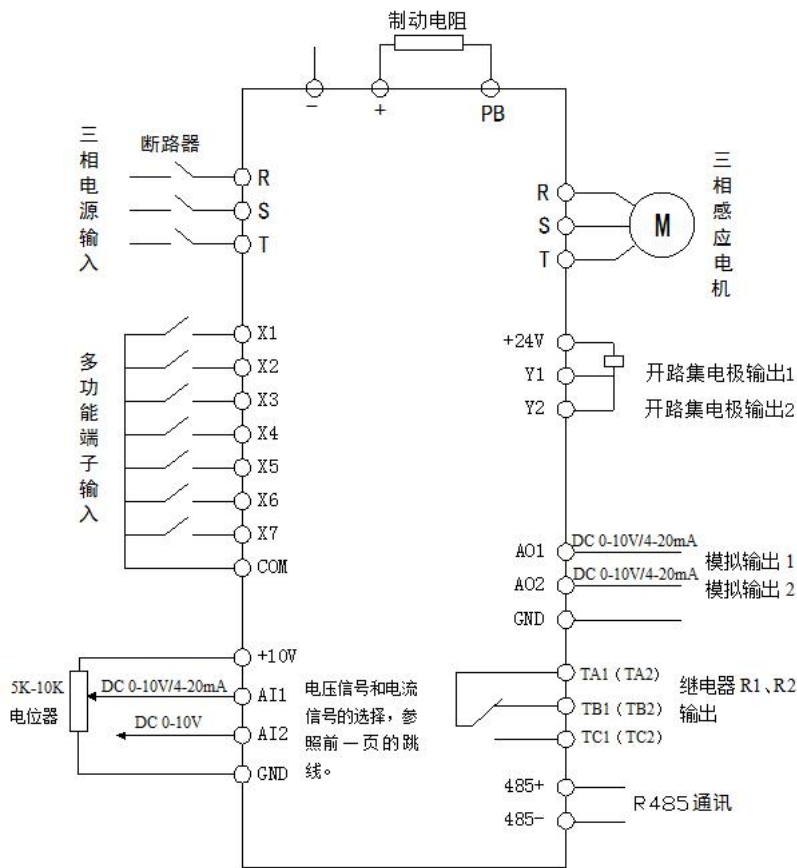
基本运行配线图
