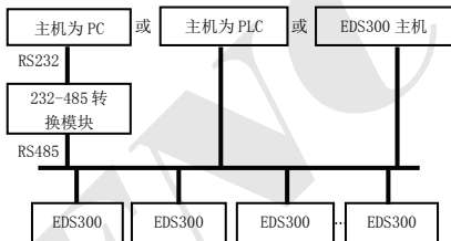
图 A-1 组网方式示意图
