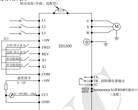
图 3-6 基本配线图
