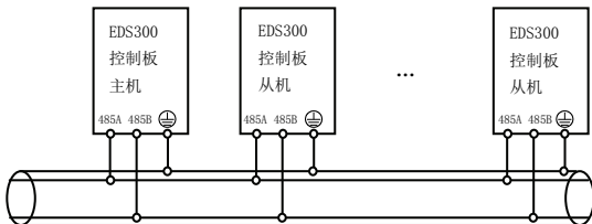
图 3-11 变频器多机通信时推荐的接线图(变频器、电机全部良好接地)
