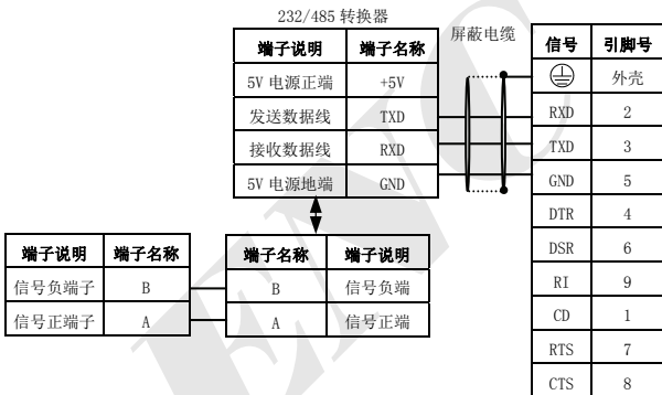
图 3-10 485 通讯配线
