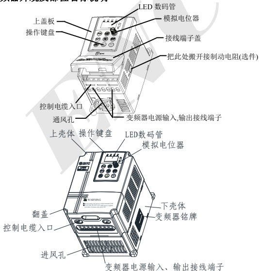
图 2-3 变频器各部位名称示意图
