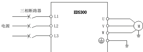
图 3-4 主回路简单配线
