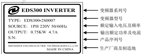
图 2-2 变频器铭牌
